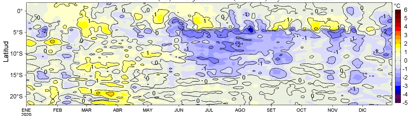
Figura 4. Variación promedio de las anomalías de la temperatura superficial del mar (TSM, °C) para una franja de 60 mn (~111 km) adyacente al litoral peruano para los últimos doce meses al 30 de diciembre de 2020. Datos: OSTIA-UKMO-L4-GLOB-v2.0 (UK Met. Office, 2012; Donlon et al, 2012) disponible en https://podaac.jpl.nasa.gov/dataset/OSTIA-UKMO-L4-GLOB-v2.0 . Las anomalías se calcularon con respecto al periodo 2007-2016. Procesamiento: LHF/AFIOF/DGIOCC.
