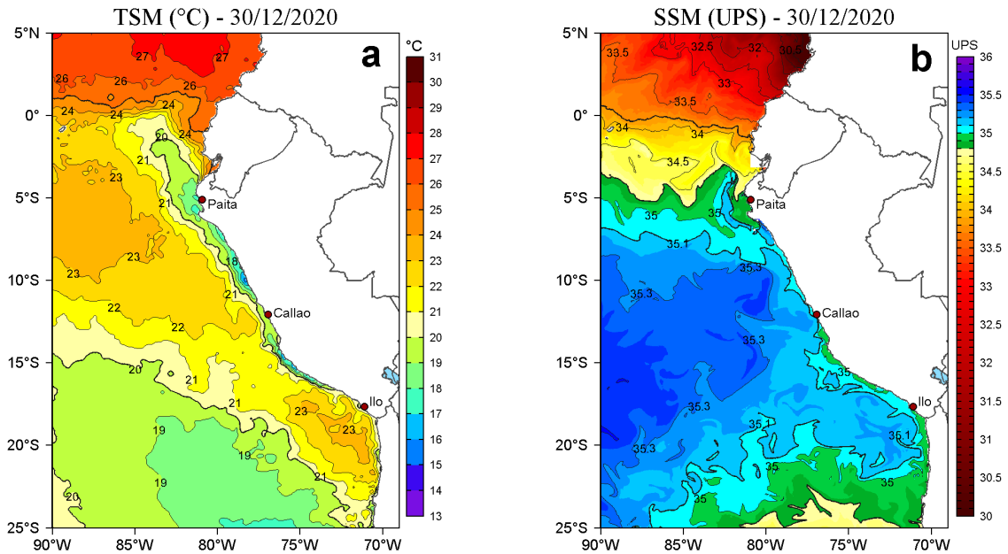
Figura 2. a) Temperatura superficial del mar (TSM, °C) y b) Salinidad superficial del mar (SSM, UPS), para el 30 de diciembre de 2020. Datos: OSTIA-UKMO-L4-GLOB-v2.0 (UK Met Office, 2012; Donlon et al, 2012) disponible en https://podaac.jpl.nasa.gov/dataset/OSTIA-UKMO-L4-GLOB-v2.0 para (a) y Hybrid Coordinate Ocean Model v. GOFS 3.1 (HYCOM; Halliwell et al., 1998; 2000; Bleck, 2001) para (b). Procesamiento: LHF/AFIOF/DGIOCC.
