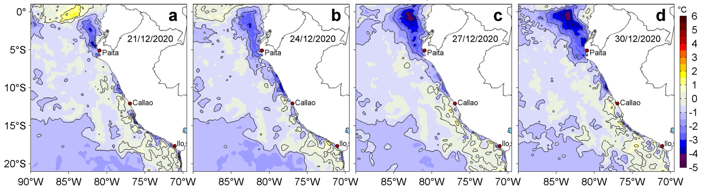
Figura 3. Anomalías de la temperatura superficial del mar (TSM, °C) para los días: a) 21, b) 24, c) 27 y d) 30 de diciembre de 2020. Las anomalías se calcularon respecto de la climatología para el periodo 2007-2016. Datos: OSTIA-UKMO-L4-GLOB-v2.0 (UK Met Office, 2012; Donlon et al, 2012). Procesamiento: LHF/AFIOF/DGIOCC.
