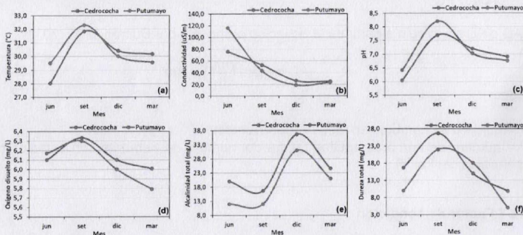
Figura 4. Variación trimestral de los principales parámetros limnológicos de laguna Cedrococha y el río Putumayo, octubre 2015-junio 2017
