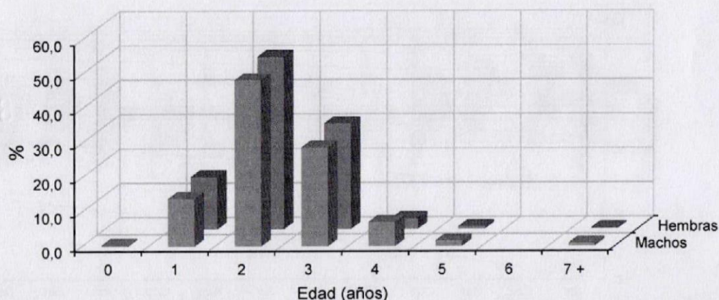
Figura 9. Composición por edades determinada para la "arahuana" Osteoglossum bicirrhosum en la cuenca del río Putumayo, oct. 2015 – jun. 2017.
