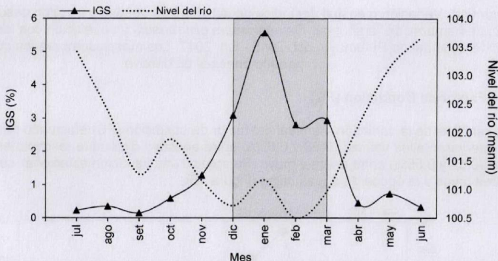
Figura 13. Variación mensual del índice gonadosomático (IGS) de hembras de "arahuana" Osteoglossum bicirrhosum y su relación con los cambios en el nivel de agua del río Putumayo, oct. 2015 - jun. 2017. Los meses sombreados corresponden al periodo principal de reproducción.
