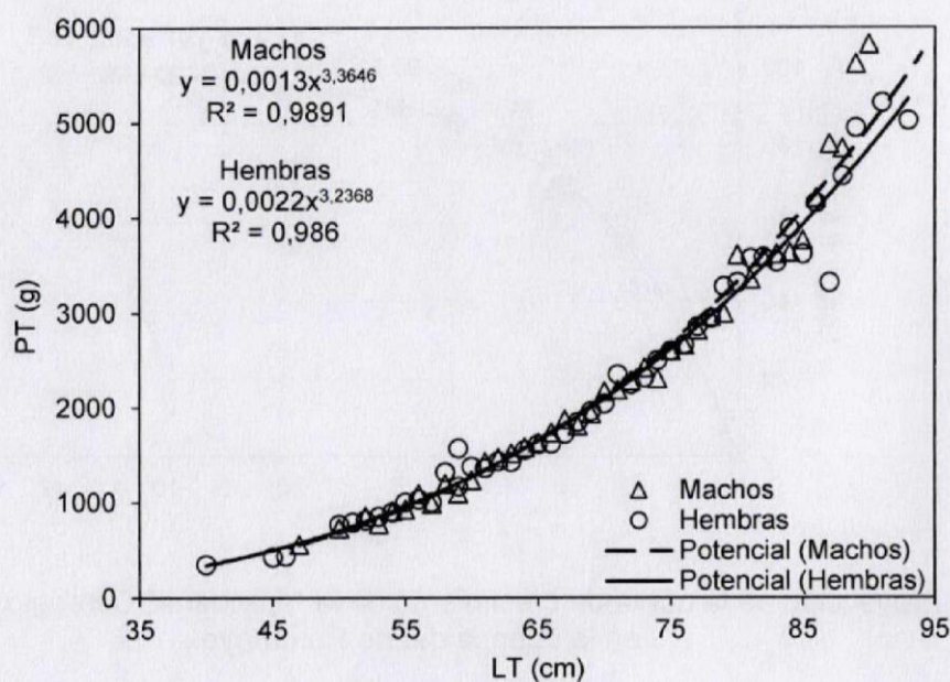
Figura 10. Relación longitud-peso determinada para la "arahuana" Osteoglossum bicirrhosum en la cuenca del río Putumayo, oct. 2015 – jun. 2017.
