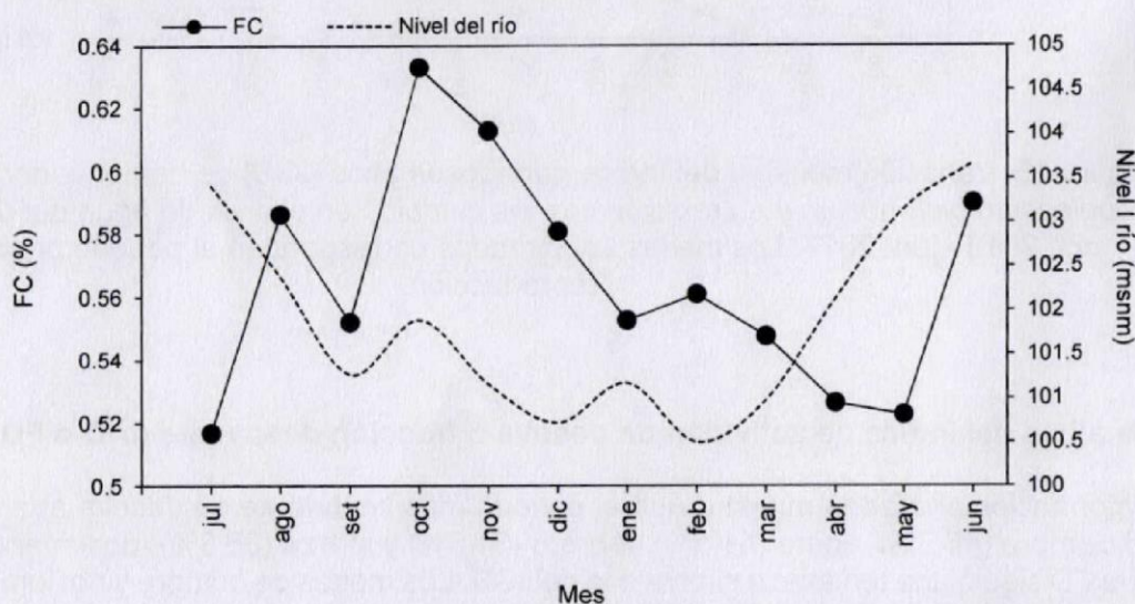
Figura 15. Variación mensual del factor de condición (determinado en hembras) de "arahuana" Osteoglossum bicirrhosum y su relación con los cambios de nivel de agua del río Putumayo, oct. 15 - jun. 17.
