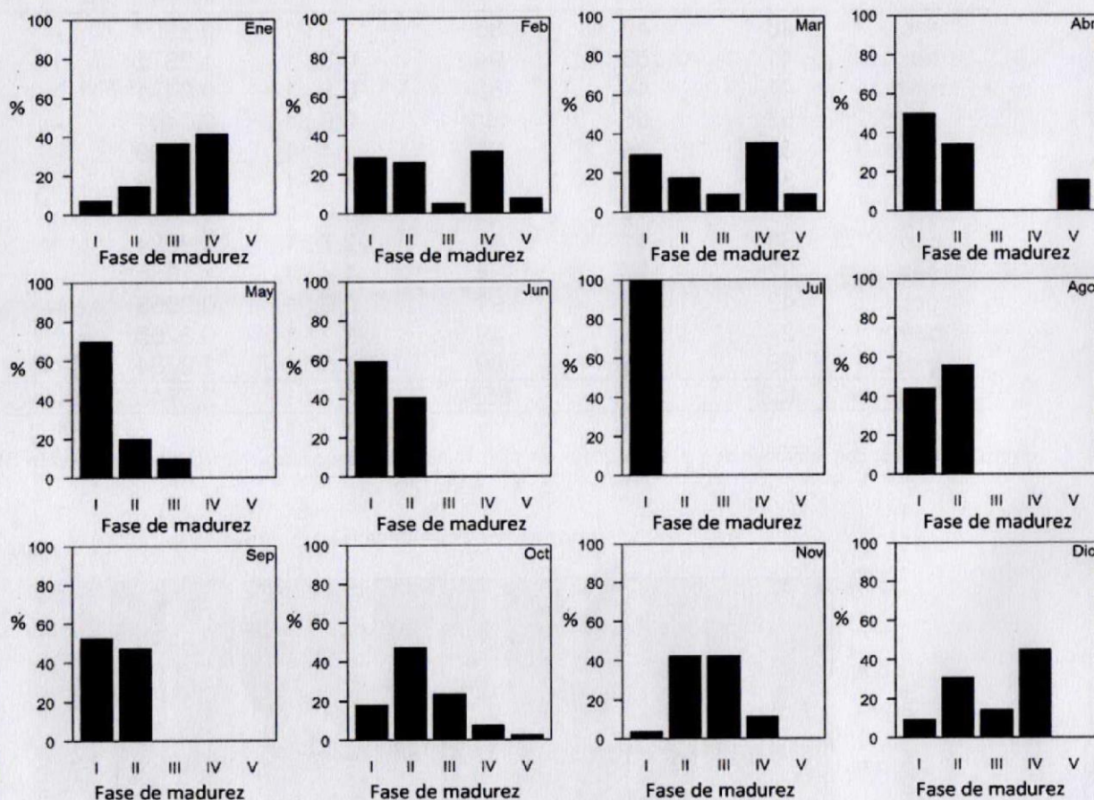
Figura 12. Evolución mensual de la madurez gonadal de hembras de "arahuana" Osteoglossum bicirrhosum en el río Putumayo en base a la escala de madurez gonadal validada histológicamente. (I: reposo; II: maduración; III: maduro; IV: desovante; V: recuperación).
