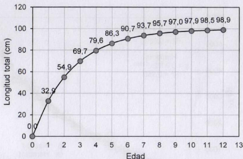
Figura 8. Proyección de la curva de crecimiento de la "arahuana" Osteoglossum bicirrhosum en la cuenca del río Putumayo.
