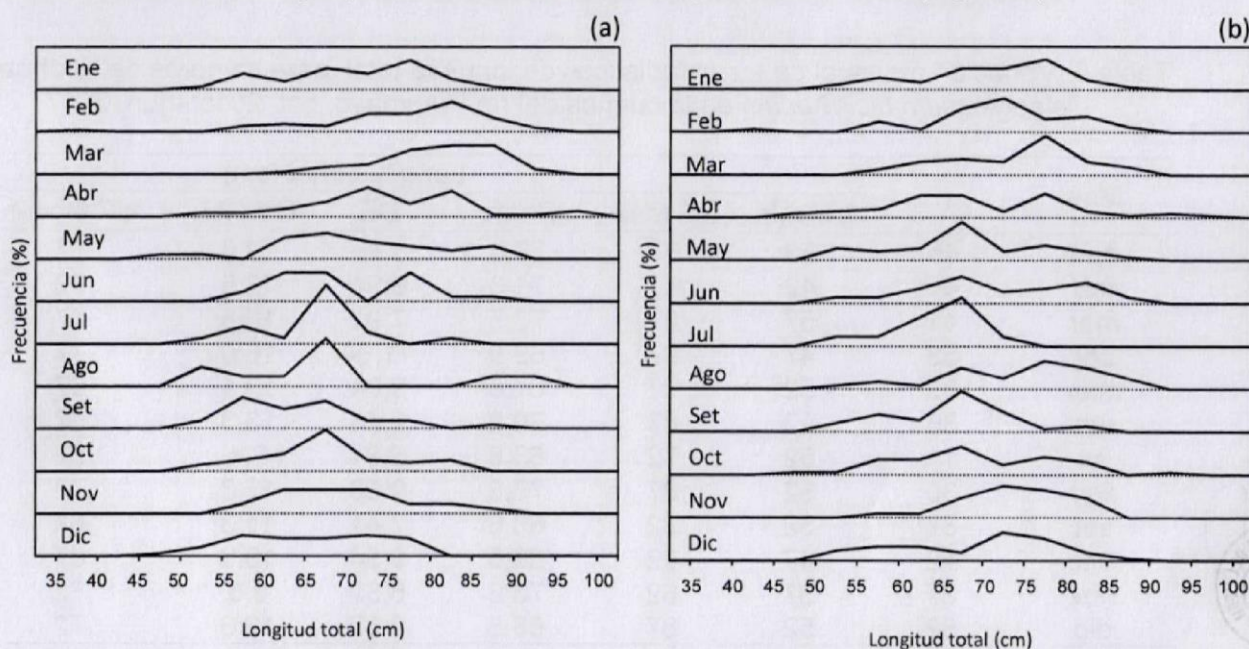
Figura 6. Variación mensual de la estructura de tallas agrupadas de "arahuana" Osteoglossum bicirrhosum en la cuenca del río Putumayo, oct. 2015 – jun. 2017 (a: Machos; b: Hembras).
