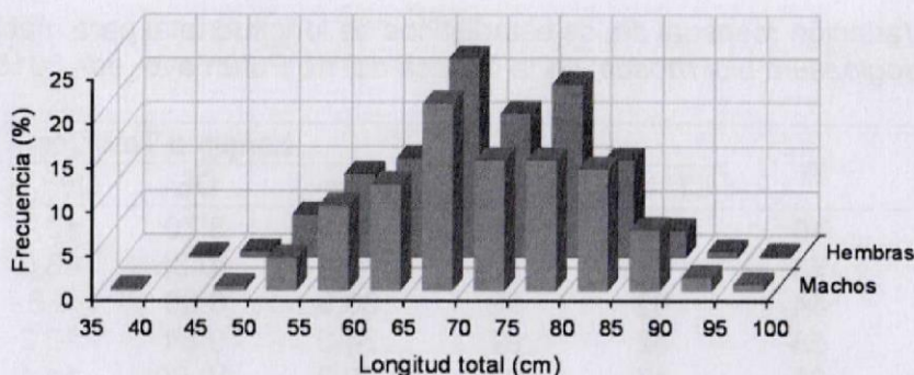
Figura 5. Estructura de tallas de hembras y machos de "arahuana" Osteoglossum bicirrhosum en la cuenca del río Putumayo, oct. 2015 – jun. 2017
