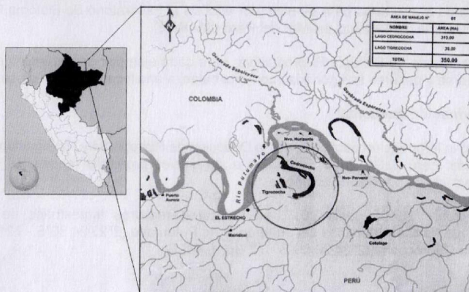
Figura 2. Ámbito de estudio: sector Cedrococha - El Estrecho - Cuenca del río Putumayo. Figura tomada de PEDICP (2013).
