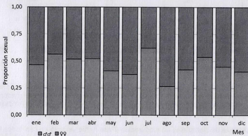
Figura 11. Proporción sexual mensual de "arahuana" Osteoglossum bicirrhosum en la cuenca del río Putumayo, oct. 2015 – jun. 2017.
