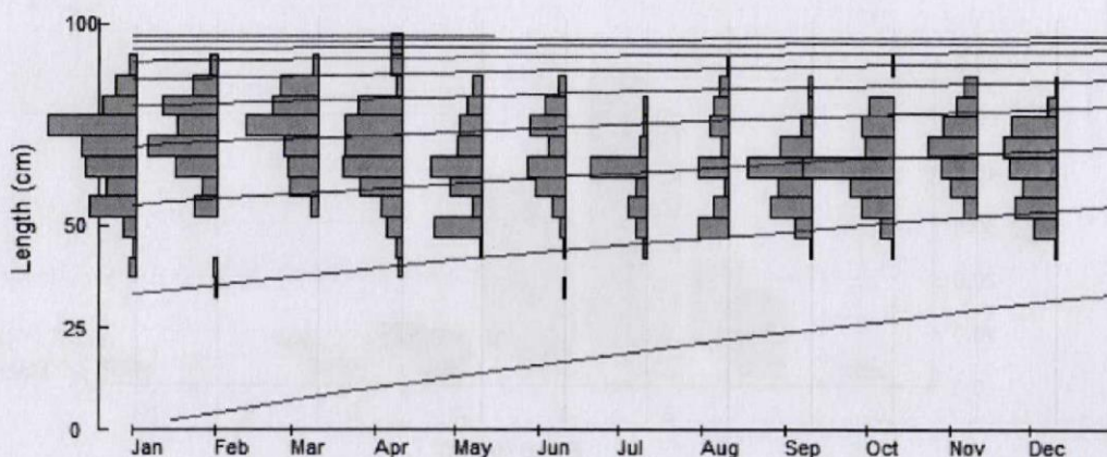
Figura 7. Histogramas de talla y curva de crecimiento determinada para la "arahuana" Osteoglossum bicirrhosum con ELEFAN en la cuenca del río Putumayo, oct. 2015 – jun. 2017.
