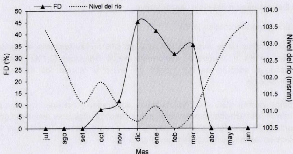
Figura 14. Variación mensual del índice de actividad de desove o fracción desovante (IAD o FD) de hembras de "arahuana" Osteoglossum bicirrhosum y su relación con los cambios de nivel de agua del río Putumayo, oct. 2015 - jun. 2017. Los meses sombreados corresponden al periodo principal de desove
